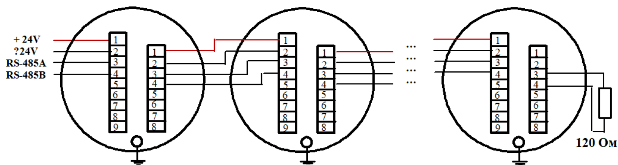
Рисунок 7 – Схема подключения ИГМ-14 по цифровому каналу RS 485.
