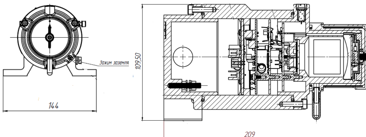
Рисунок 4 – Габаритные размеры ИГМ-14 (корпус тип 5)
