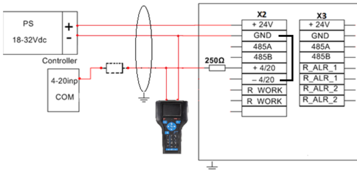
Рисунок 8 – Схема подключения ИГМ-14 по 4-20 Ма (трехпроводная схема).
