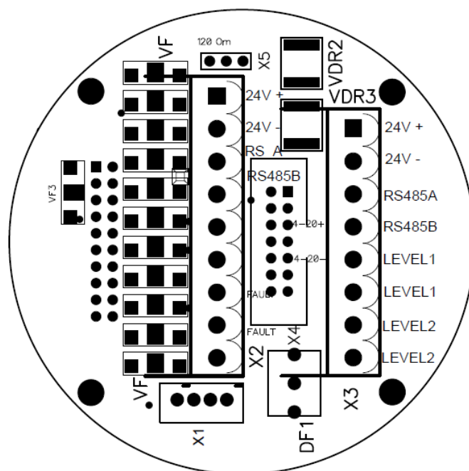
Рисунок 10 – Расположение и назначение клемм, используемых при монтаже.
