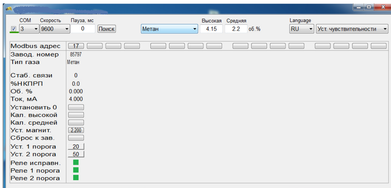
Рис.6 Интерфейс сервисной программы ИГМ-14
