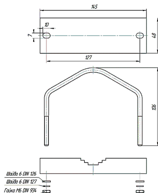
Рисунок 6 – Крепёжная скоба и внешний вид смонтированного на трубу прибора
